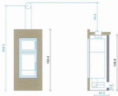
Verbreiterungsstutzenrohr 185 mm DM
